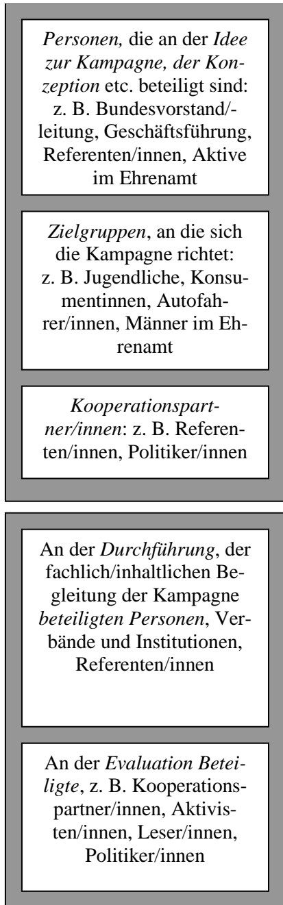
Abbildung 3: Gendersensible Prozessschrittanalyse
