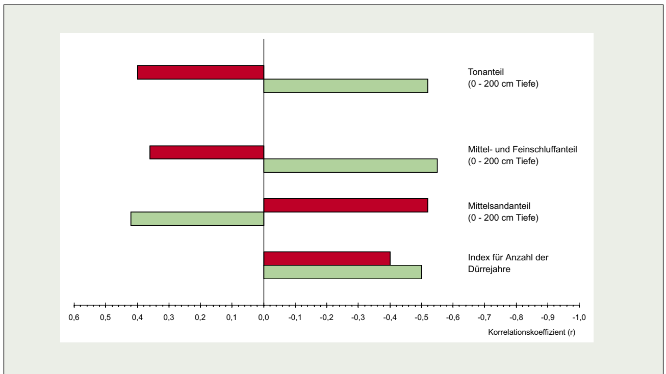
Abb. 7: Signifikante Korrelationen zwischen Standortmerkmalen und der Höhenwuchsleistung der Stieleiche (■ Tf-Tm, K2) und Traubeneiche (■ Tm-Tt, M2-Z2)
