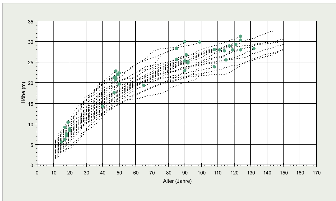
Abb. 5: Höhenwachstum und Höhenentwicklung der Stieleiche auf Standorten der ökologischen Wuchsreihe „gutwüchsige Stieleiche (SEI I)“
