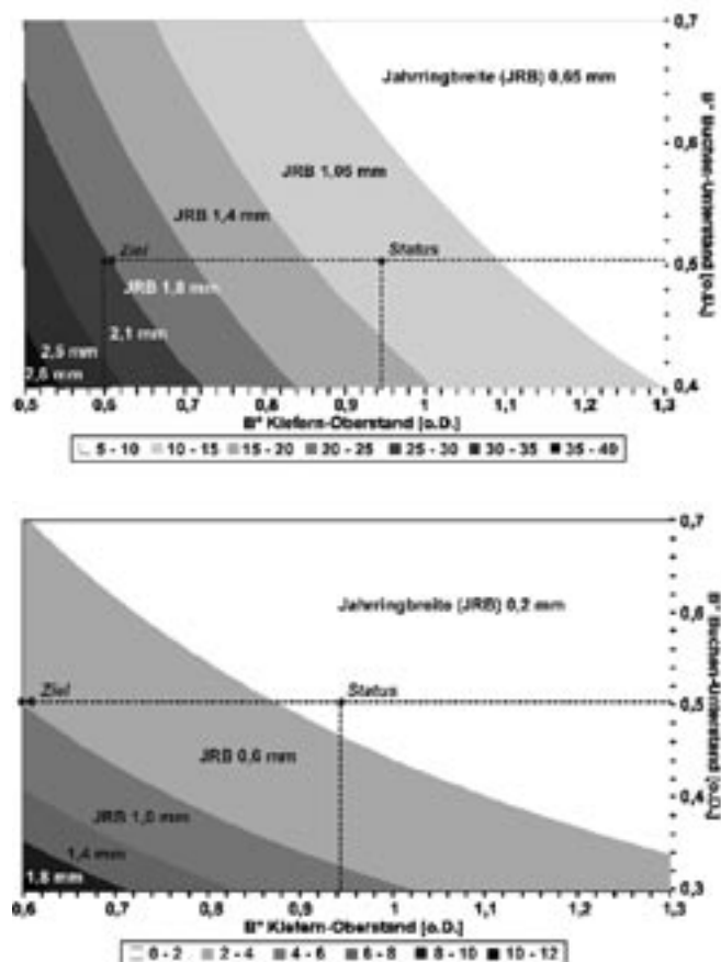
Abb. 16 und 17: Nomogramme zur Darstellung des Kreisflächenzuwachses des Bestandesmittelbaumes von Oberstandskiefern (oben) und Unterstandsbuchen (unten) in Abhängigkeit von den Bestockungsgraden des Kiefern-Ober- und des Buchen-Unterstandes am Beispiel der Mischbestandsfläche IV
