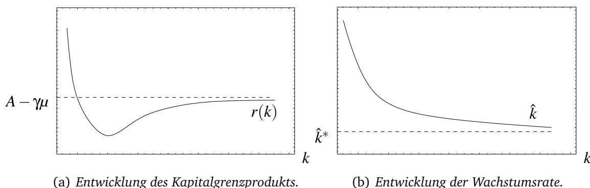
Abbildung 2: Die Anpassungsdynamik.
