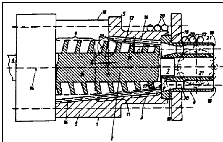
Abbildung 3: Extruder und Matrice gem. Patent von Tessmer
